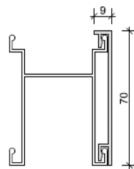
J1 RODAPÉ DUPLO ESCALA: 1/20
