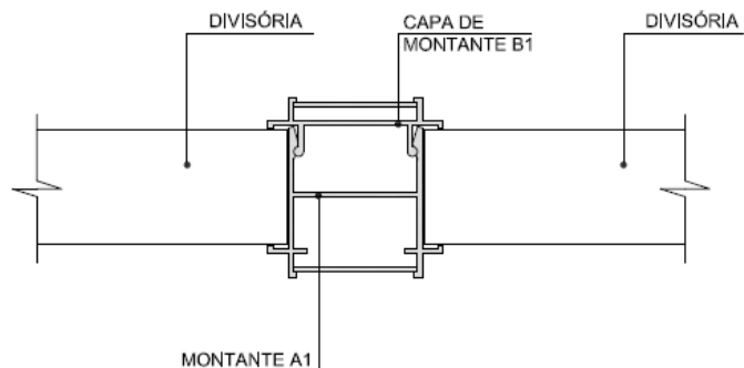
K1 DETALHE MONTANTE ENTRE 2 DIVISÓRIAS ESCALA: 1/20
