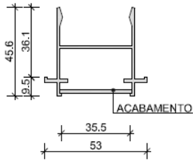
A1 MONTANTE ESCALA: 1/20
