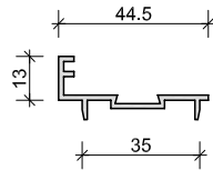
E1 BATENTE DE PORTA ESCALA: 1/20
