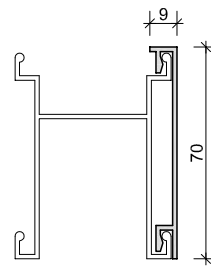
J1 RODAPÉ DUPLO ESCALA: 1/20
