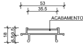
B1 CAPA DE MONTANTE ESCALA: 1/20
