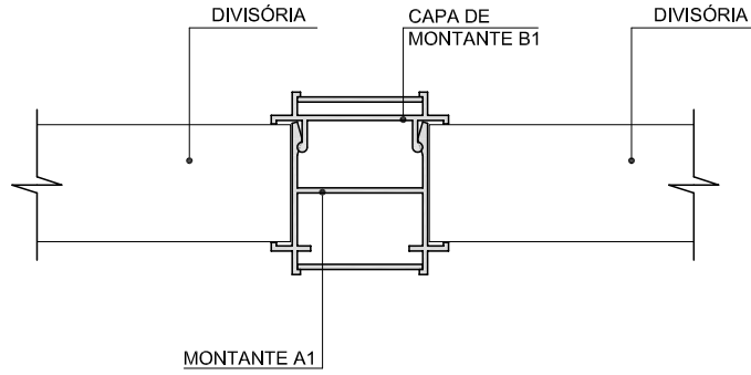
K1 DETALHE MONTANTE ENTRE 2 DIVISÓRIAS ESCALA: 1/20
