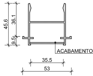
A1 MONTANTE ESCALA: 1/20
