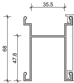
I1 MACACO ESCALA: 1/20
