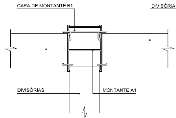
L1 DETALHE MONTANTE ENTRE 3 DIVISÓRIAS ESCALA: 1/20
