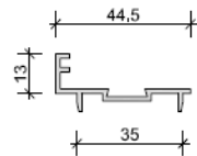
E1 BATENTE DE PORTA ESCALA: 1/20
