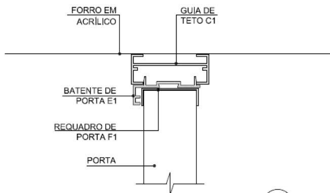
R1 DETALHE ENCONTRO PORTA/FORRO ESCALA: 1/20
