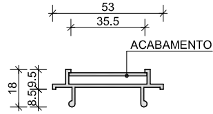
B1 CAPA DE MONTANTE ESCALA: 1/20
