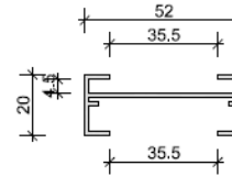
C1 GUIA DE TETO ESCALA: 1/20
