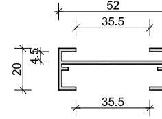
C1 GUIA DE TETO ESCALA: 1/20
