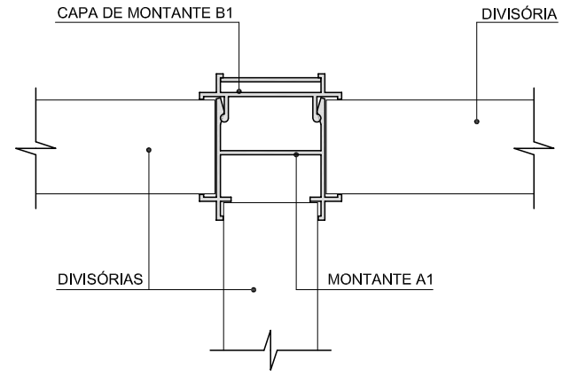
L1 DETALHE MONTANTE ENTRE 3 DIVISÓRIAS ESCALA: 1/20
