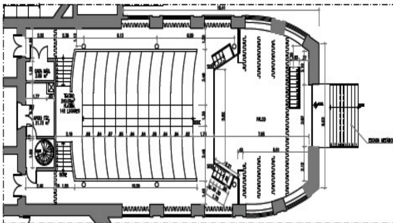
TÉRREO-TEATRO/EXECUTIVO ESCALA: 1/100
