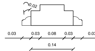
CORTE ADUELA E ALIZAR 3º PAVIMENTO
