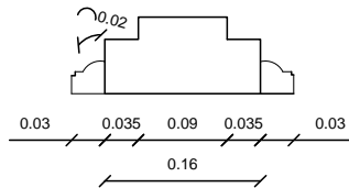
CORTE ADUELA E ALIZAR TÉRREO FEMININO
